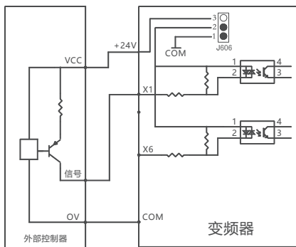
图 4.15 PNP 型接线图
