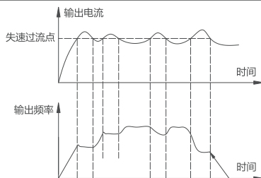
图 8-7-1 过流失速动作示意图
