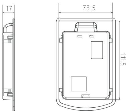
图 5.7 托板的外形尺寸
