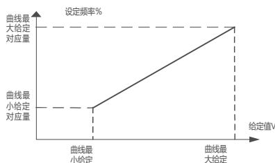
图 8-2-1 AI 曲线 1 设定
