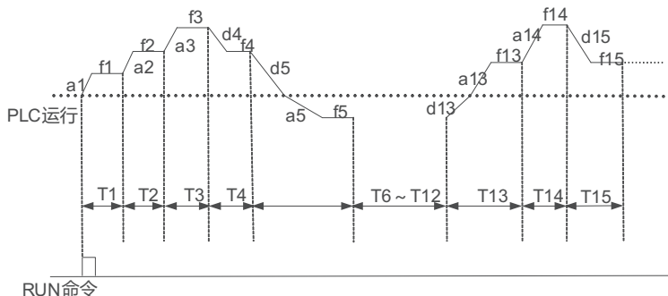
图 8-2-5 简易 PLC 单循环后保持最终值方式
