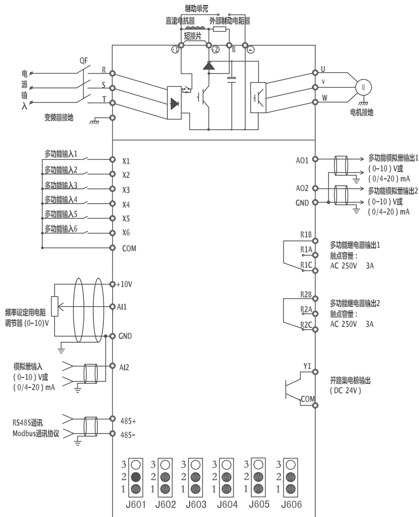
图 4.12 NVF2G-1.5/PS4 ~ NVF2G-400/TS4(-L) 接线图
