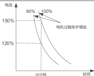
图 8-9-1 电机过载反时限曲线示意图
