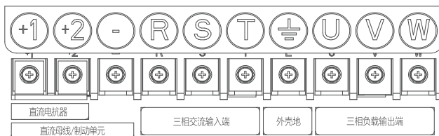
图 4.8 主回路端子 NVF2G-45/TS4~110/PS4
