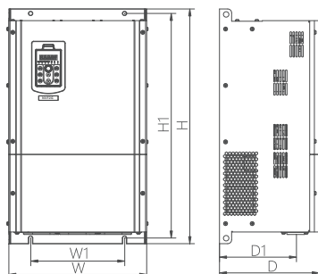
图 5.3 NVF2G-30/TS4~ NVF2G-75/PS4外形和安装尺寸图
