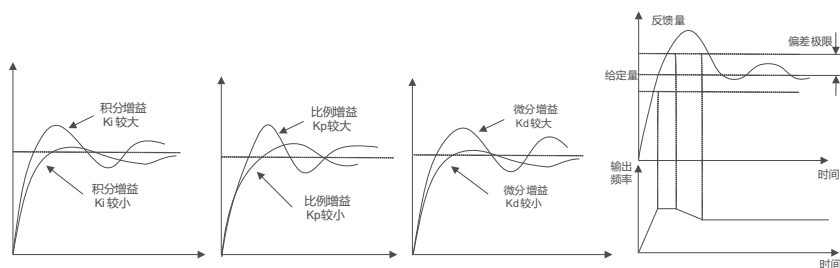
图 8-2-8 过程 PID 参数影响示意
