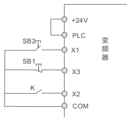
图 8-1-4 三线制控制模式 2
