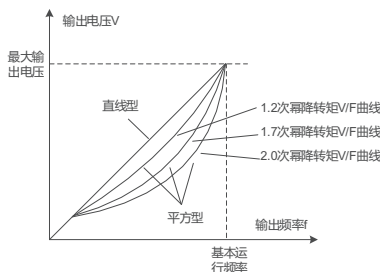
图 8-5-3 降转矩 V/F 曲线
