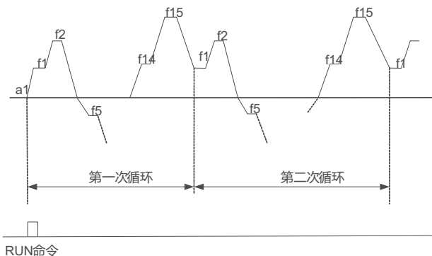
图 8-2-6 简易 PLC 连续循环方式
