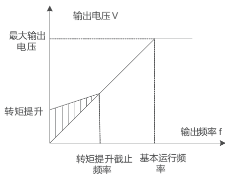
图 8-5-1 通用恒转矩直线 V/F 曲线
