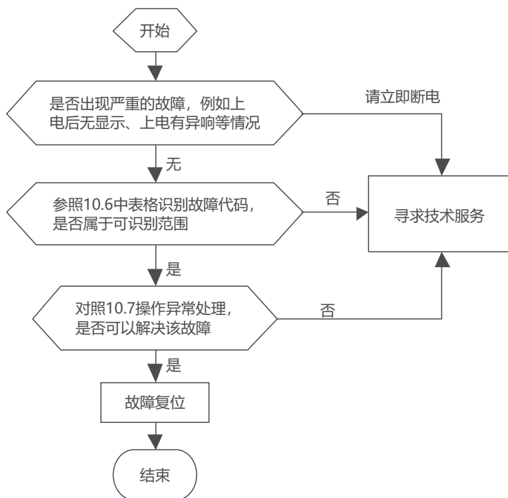
图10.2 故障诊断流程图
