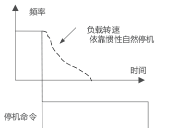
图 8-3-5 自由停机时序图
