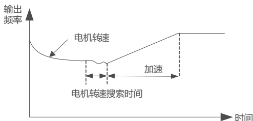
图 8-3-3 转速追踪再启动时序图
