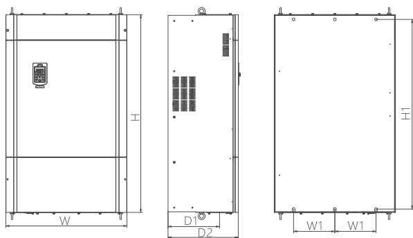
图 5.5 NVF2G-315/TS4-L~ NVF2G-400/TS4-L外形和安装尺寸图
