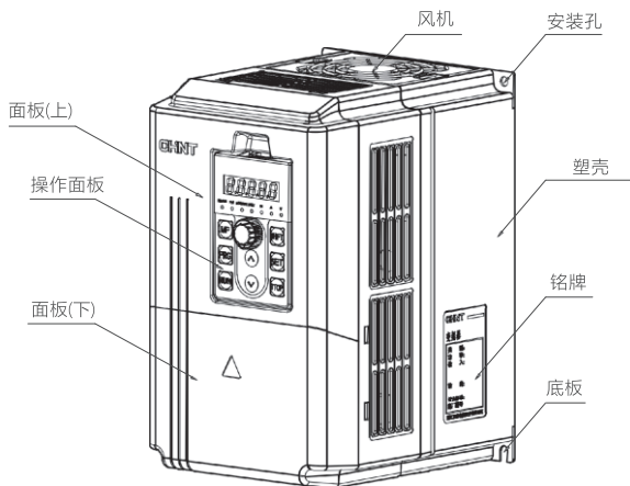
图 4.1 NVF2G-1.5/PS4~NVF2G-11/PS4外形部件图
