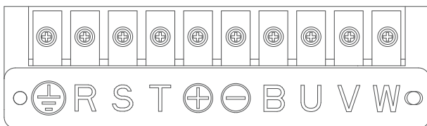
图 4.6 主回路端子 NVF2G-1.5/PS4~30/PS4
