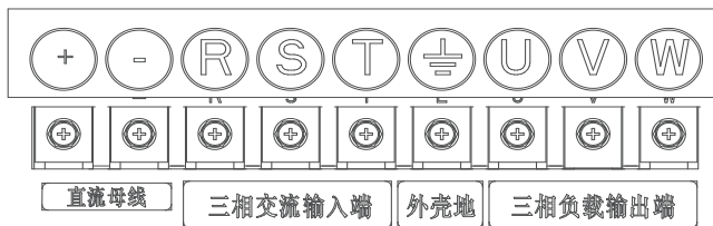
图 4.7 主回路端子 NVF2G-30/TS4~45/PS4
