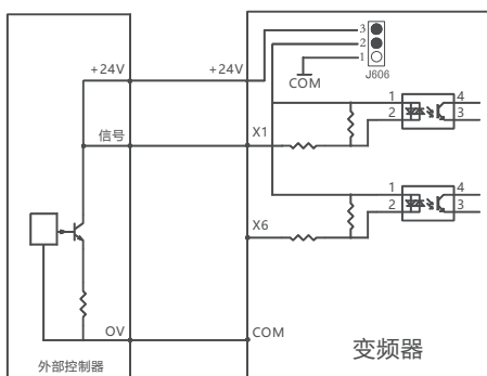
图 4.16 NPN 型接线图
