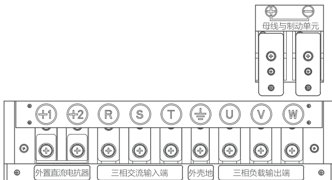
图 4.10 主回路端子 NVF2G-160/TS4(-L)~315/PS4(-L)
