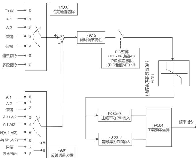
图 8-2-7 过程 PID 作为主频率示意图
