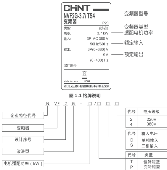
图 1.1 铭牌说明和产品型号命名规则
