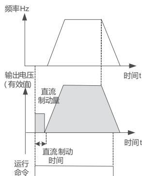
图 8-3-2 先制动再启动时序图
