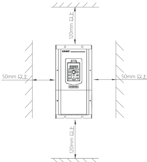
图 2.1 变频器安装示意图
