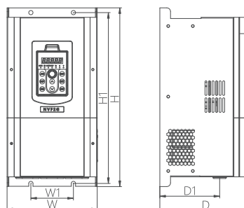
图 5.2 NVF2G-11/TS4~ NVF2G-30/PS4外形和安装尺寸图
