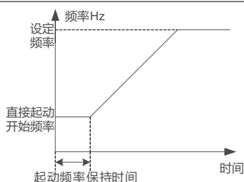
图 8-3-1 直接启动时序图
