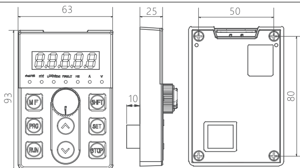
图 5.6 显示盒外形尺寸
