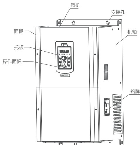
图 4.3 NVF2G-30/TS4~NVF2G-75/TS4外形部件图
