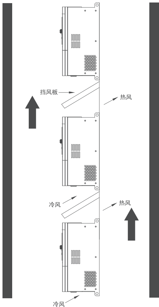
图 2.2 多台变频器垂直安装
