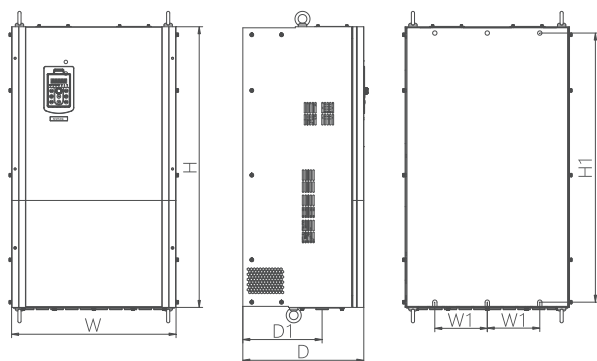
图 5.4 NVF2G-75/TS4~ NVF2G-315/PS4(-L)外形和安装尺寸图
