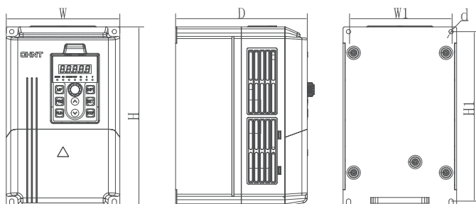
图 5.1 NVF2G-1.5/PS4~ NVF2G-11/PS4外形和安装尺寸图
