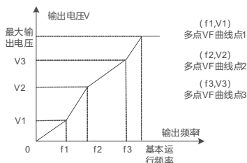
图 8-5-2 自定义多点 V/F 曲线
