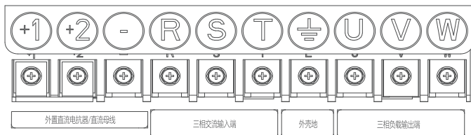
图 4.9 主回路端子 NVF2G-110/TS4(-L)~160/PS4(-L)
