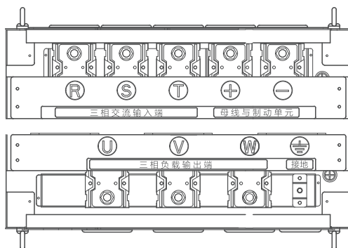
图 4.11 主回路端子 NVF2G-315/TS4-L~400/TS4-L
