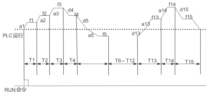
图 8-2-4 简易 PLC 单循环后停机方式
