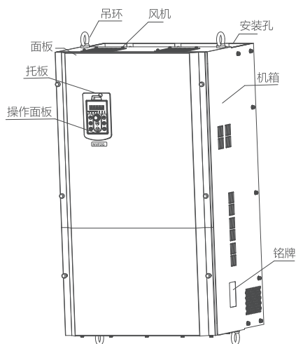
图 4.4 NVF2G-75/TS4~NVF2G-315/PS4(-L)外形部件图
