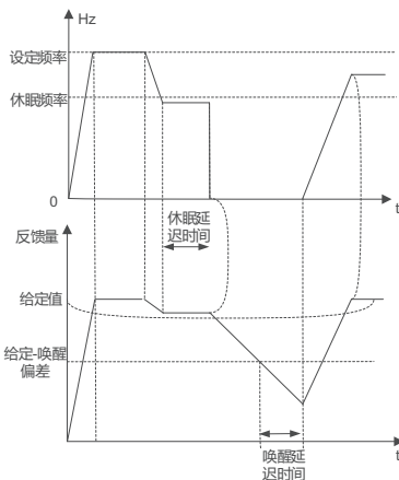
图 8-21-1 休眠与唤醒示意图
